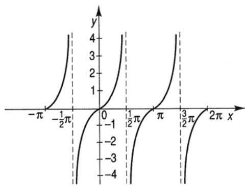
y = \operatorname{tg}x
