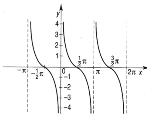
y = \operatorname{ctg}x
